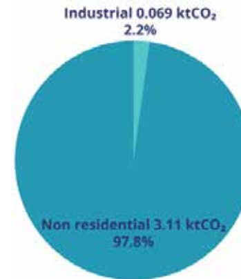
Fíor 4.9 Astaíochtaí neamhchónaitheacha agus tionsclaíocha sa CD. 2019
