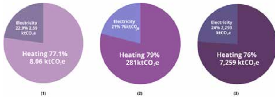
Fíor 4.4 Crios Dícharbónaithe (1), Contae Dhún na nGall (2) agus Scoilt Náisiúnta (3) d'astaíochtaí CO 2 fuinneamh cónaitheach
