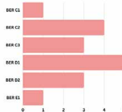
Fíor 4.18. Dáileadh BER Intire n
