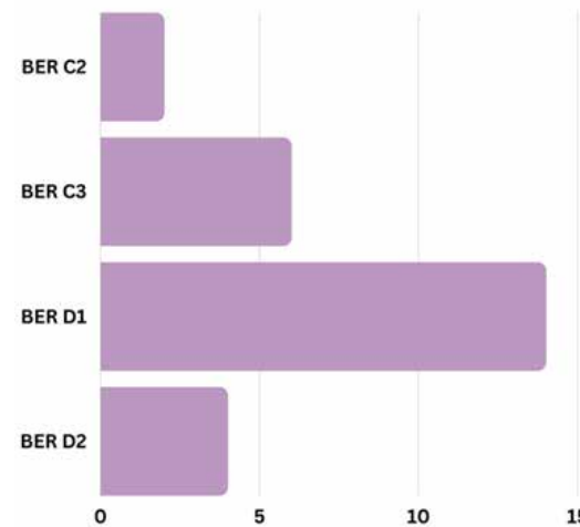
Fíor 4.6. Dáileadh BER Intíre
