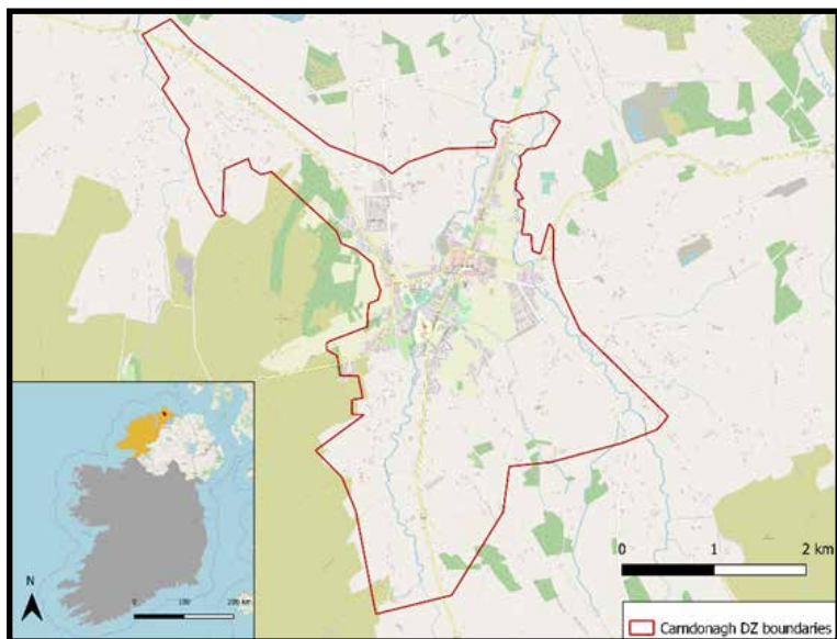
Fíor 4.14 Léarscáil de Chrios Dícharbónaithe Charn Domhnach
