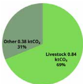
Fíor 4.23 Miondealú ar astaíochtaí talmhaíochta sa CD, 2019
