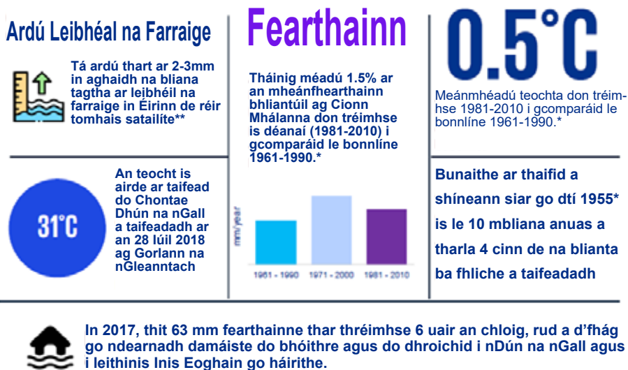
Fíor 2.1 – Buaicphointí maidir leis an Athrú Aeráide atá Sainaitheanta d'Éirinn agus do Dhún na nGall Foinse: KPMG, Measúnú Riosca Chomhairle Contae Dhún na nGall ar Athrú Aeráide, 2023.
