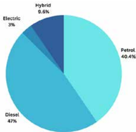
Fíor 4.20 Miondealú carranna príobháideacha de réir an chineáil breosla sa CD. 2016
