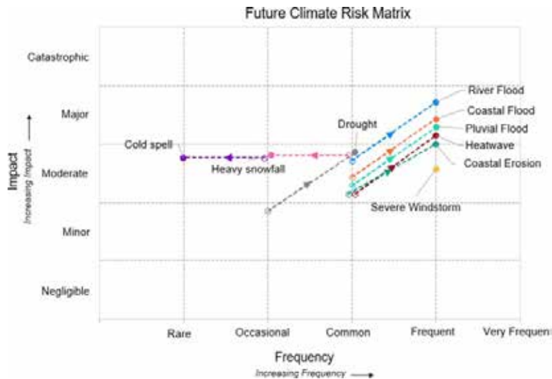
Fíor 2.3 Maitrís Riosca Aeráide amach anseo do Chontae Dhún na nGall (Foinse, KPMG Measúnú Riosca Chomhairle Contae Dhún na nGall ar Athrú Aeráide, 2023).
