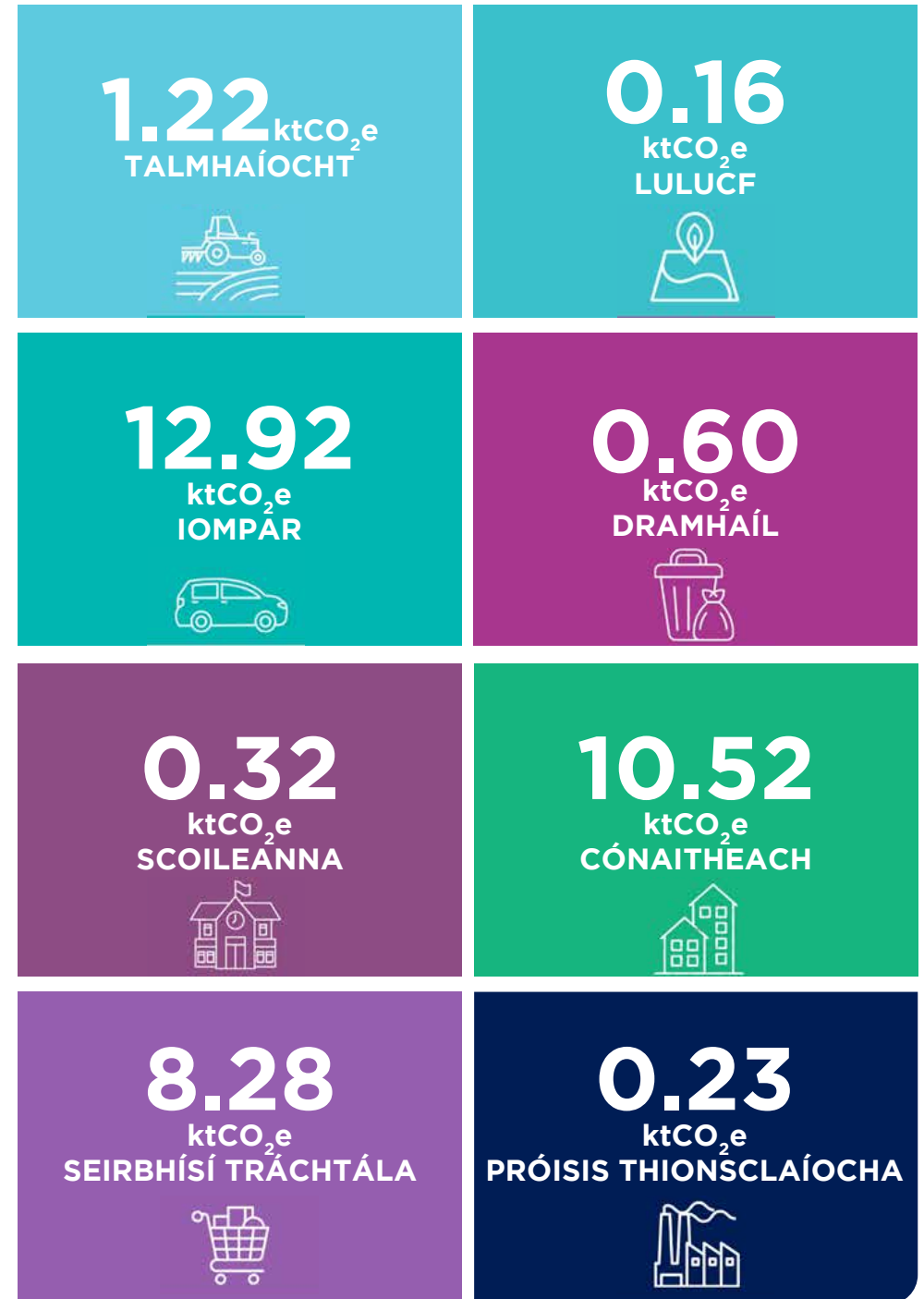
Fíor 4.15 Torthaí Fhardail Astaíochtaí Bonnline 2019 - Charn Domhnach
