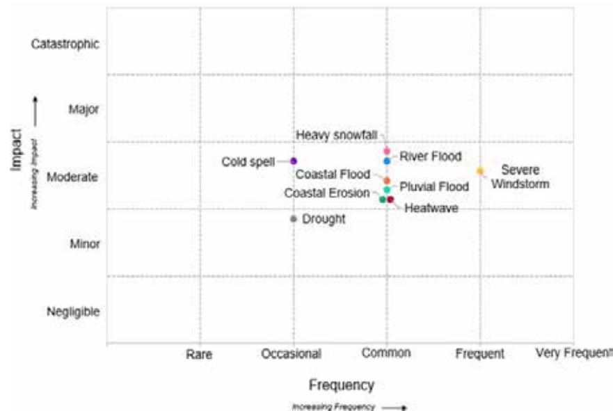
Fíor 2.2: Maitrís Riosca Aeráide Reatha do Chontae Dhún na nGall (Foinse, KPMG Measúnú Riosca Chomhairle Contae Dhún na nGall ar Athrú Aeráide, 2023)
