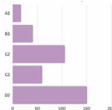
Fíor 4.22 Dáileadh na bhfoirgneamh thráchtála ag brath ar rátáil RFF sa CD
