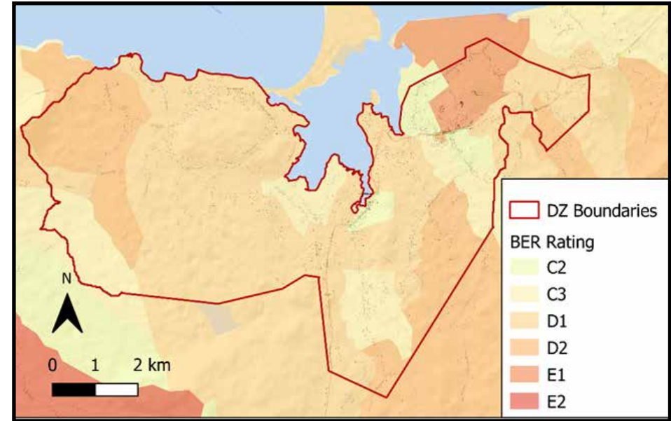
Fíor 4.5 Meánráta BER Cónaitheach in aghaidh an cheantair bhig sa CD
