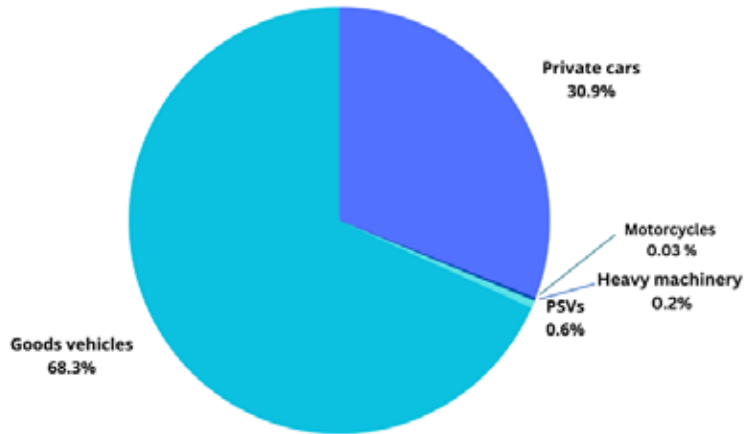
Fíor 4.19 Miondealú ar astaíochtaí iompair do gach cineál feithicle
