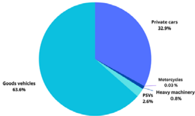
Fíor 4.7 Miondealú ar astaíochtaí iompair do gach cineál feithicle
