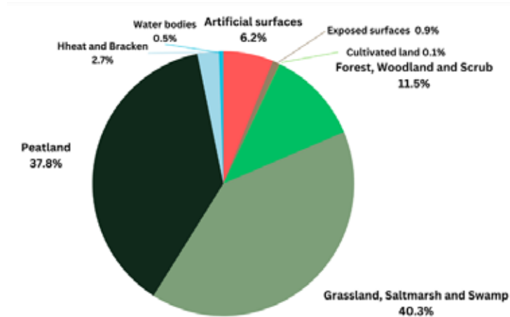
Fíor 4.13 Úsáid Talaimh sa CD. 2019
