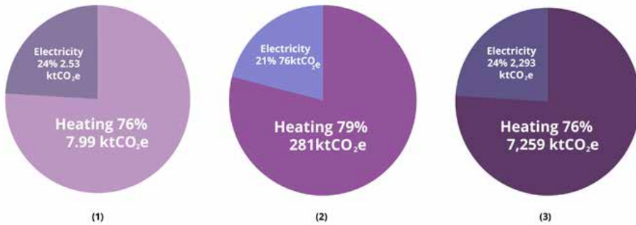
Fíor 4.16 Críos Dícharbónaithe (1), Contae Dhún na nGall (2) agus Scoilt Náisiúnta (3) d'astaíochtaí CO 2 fuinneamh cónaitheach
