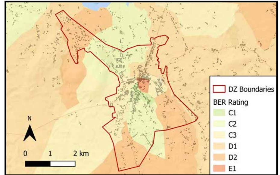
Fíor 4.17 Meánráitil BER Chónaitheach in aghaidh an cheantair bhig sa CD
