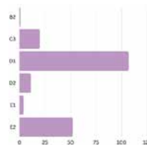
Fíor 4.10. Dáileadh foirgneamh thráchtála ag brath ar rátáil BER sa CD
