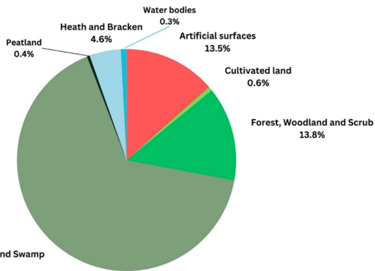
Fíor 4.25 Limistéar úsáid talaimh sa CD.2019
