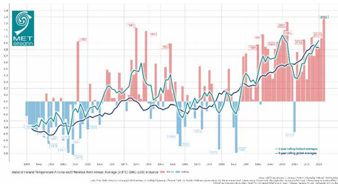
Fíor 1.2 Oileán na hÉireann 1900-2022 Aimhrialtachtaí Teochta (°C) (difríocht ó 1961-1990) (Foinse Met Éireann)
