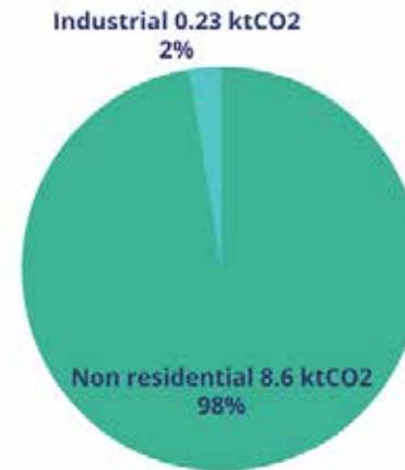
Fíor 4.21 Astaíochtaí neamhchónaitheacha agus tionsclaíocha sa CD. 2019
