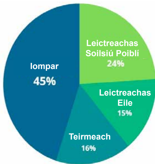
Fíor 2.6: Astaíochtaí GCT Chomhairle Contae Dhún na nGall
