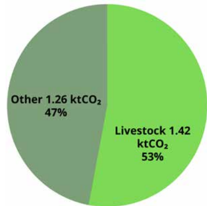
Fíor 4.11 Miondealú ar astaíochtaí talmhaíochta sa CD. 2019
