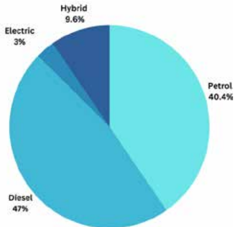
Fíor 4.8 Miondealú carranna príobháideacha de réir an chineáil bhreosla sa CD. 2016
